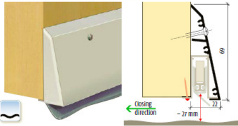
Socket mit | Socle avec | Socle with → Planet RF
