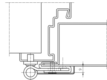
steel door
