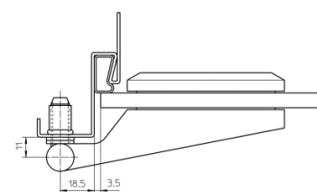
Rahmenteil oben
