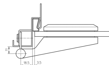
Rahmenteil unten
