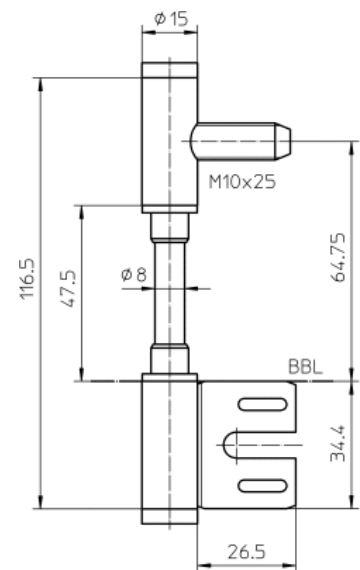
Vorderansicht
