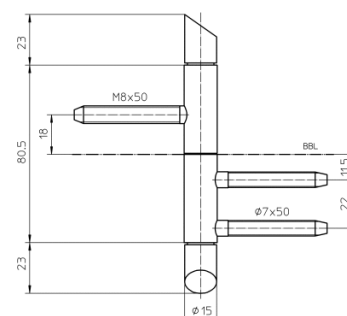
Vorderansicht
