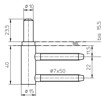
Vorderansicht
