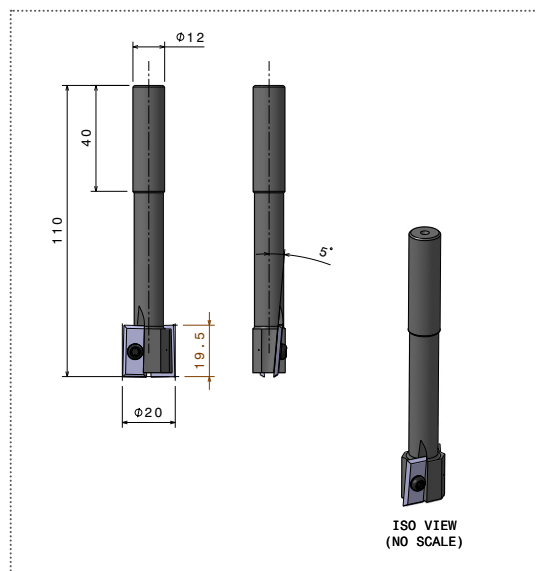
FRESA / MILLING TOOL N.1
