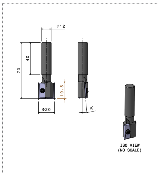
FRESA / MILLING TOOL N.2
