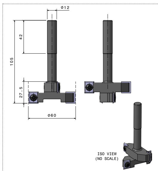
FRESA / MILLING TOOL N.3
